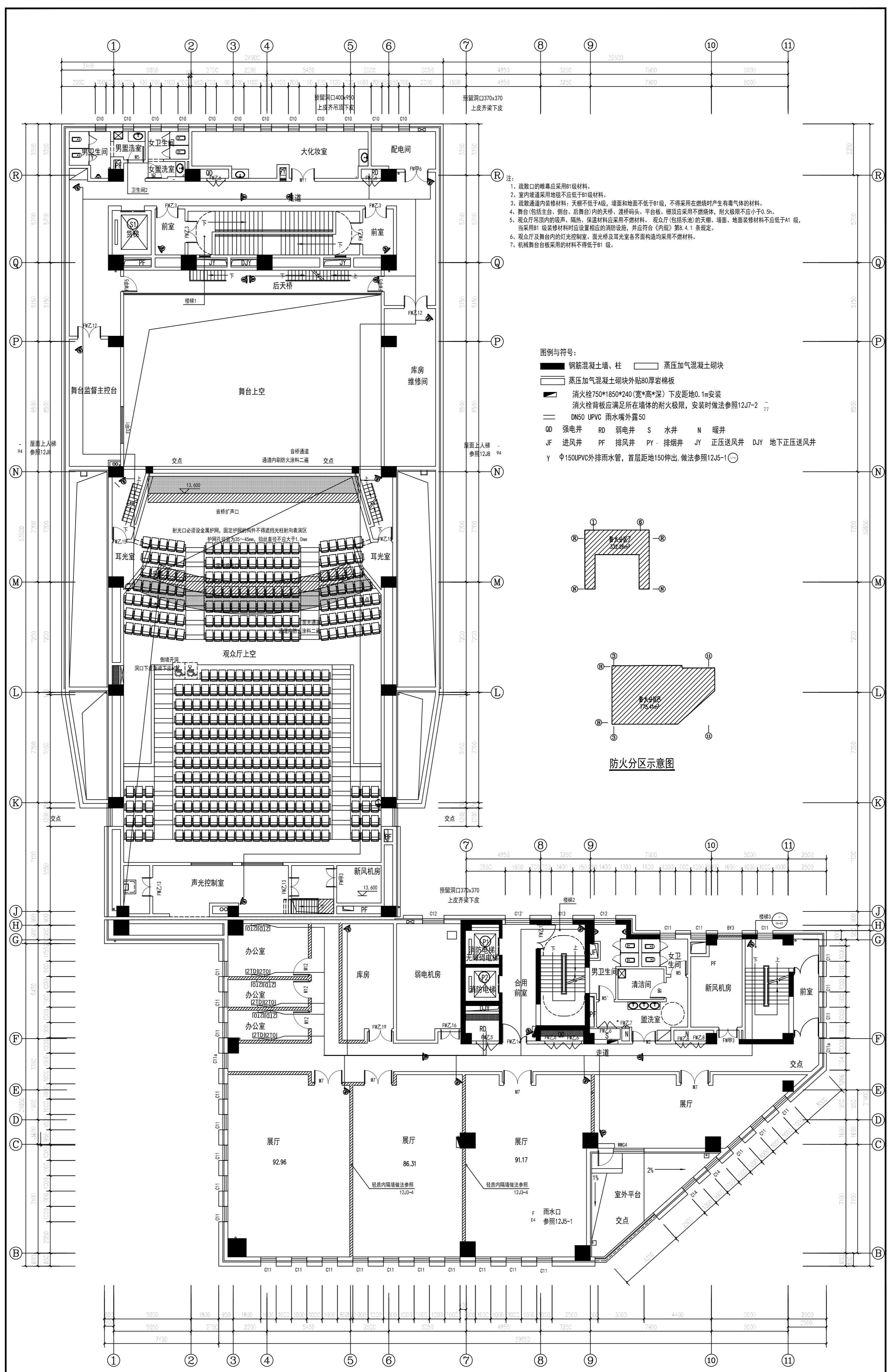
四层平面图 1:100 四层建筑面积: 1148.5m 2
