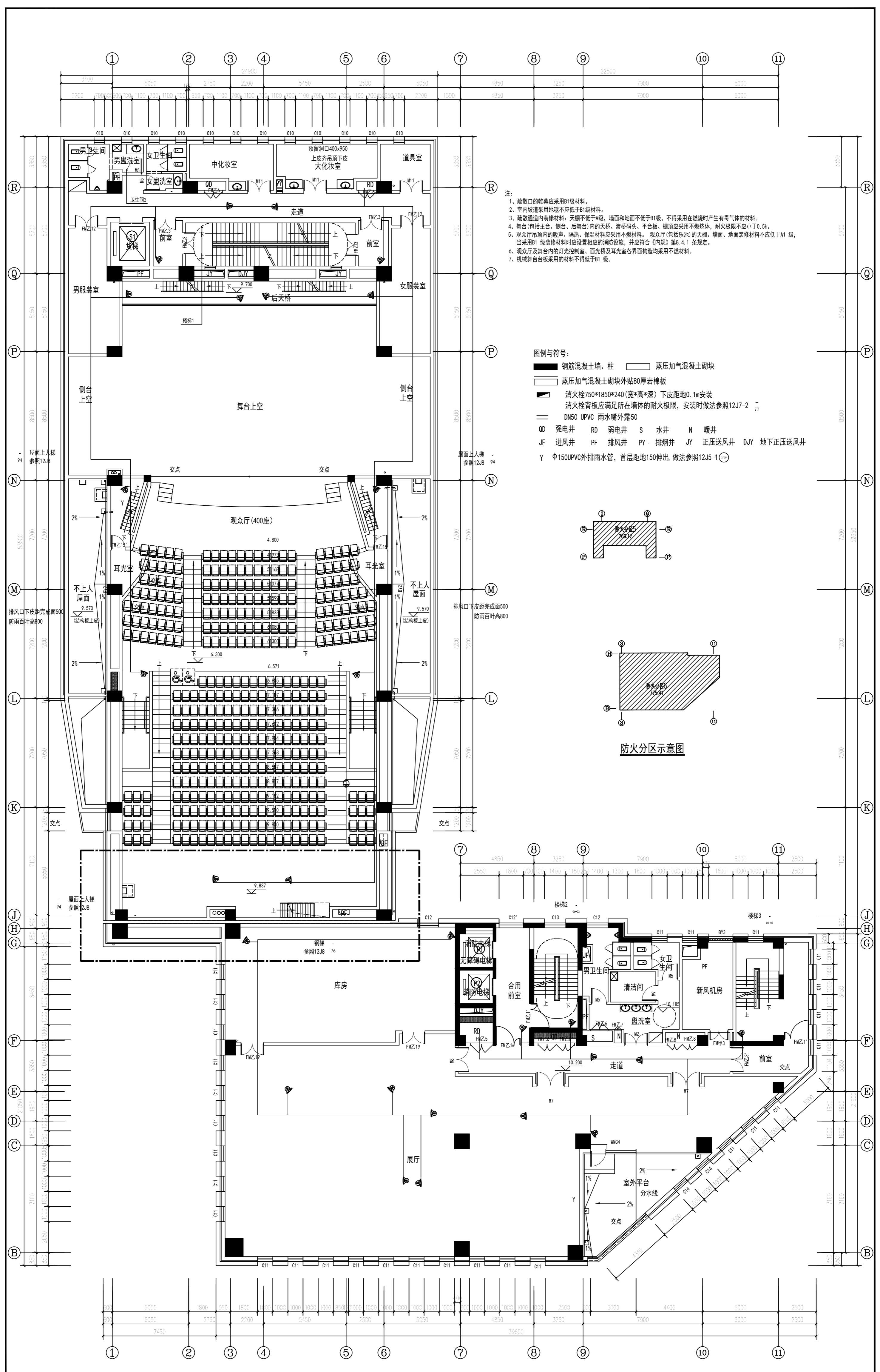
三层平面图 1:100
